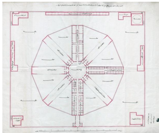
Şekil 7: Ferik Blunt Paşa mühürlü ışınsal planlı hapishane projesi (BOA, Plan-Proje-Kroki, Plan-Projeler [PLK. p.], No: 5384).
