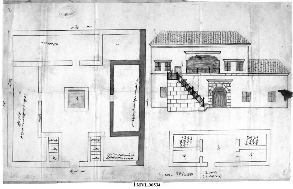
Şekil 1: 1865 Tarihli Ankara Hapishane Projesi (BOA, İ. MVL. No. 534, Gömlek No. 23980).
