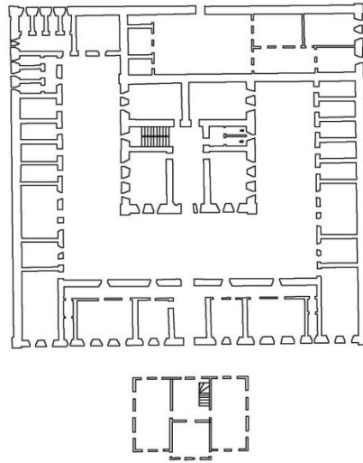
Şekil 2: 1897 Tarihli Ankara Hapishane Projesi (, BEO, No. 908, Gömlek No. 68047 adlı dosyadan düzenlenmiştir).
